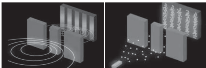
Рис. 1. Електрон – хвиля
