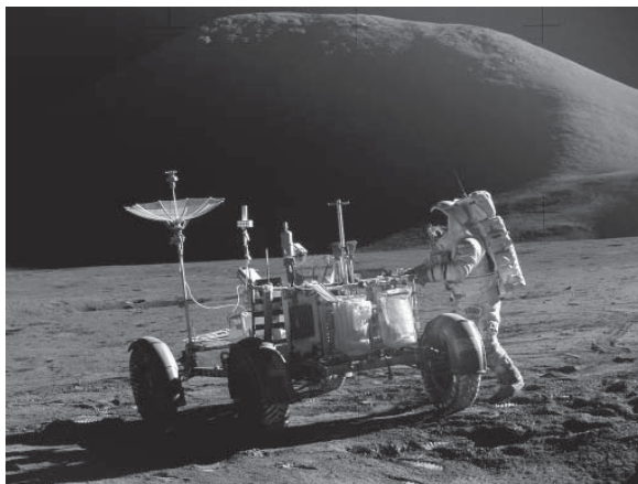
Фото 1. На поверхні Місяця, фото NASA
