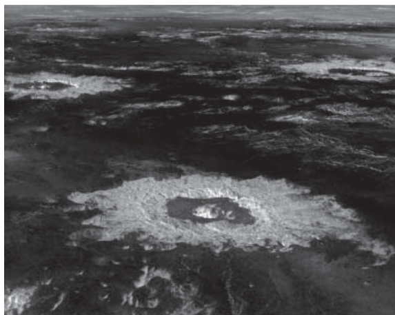
Фото 2. На поверхні Венери, фото міжпланетної станції «Магеллан»
