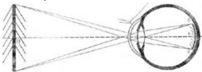
Рис. 2. Схема утворення зображення на сітківці ока
